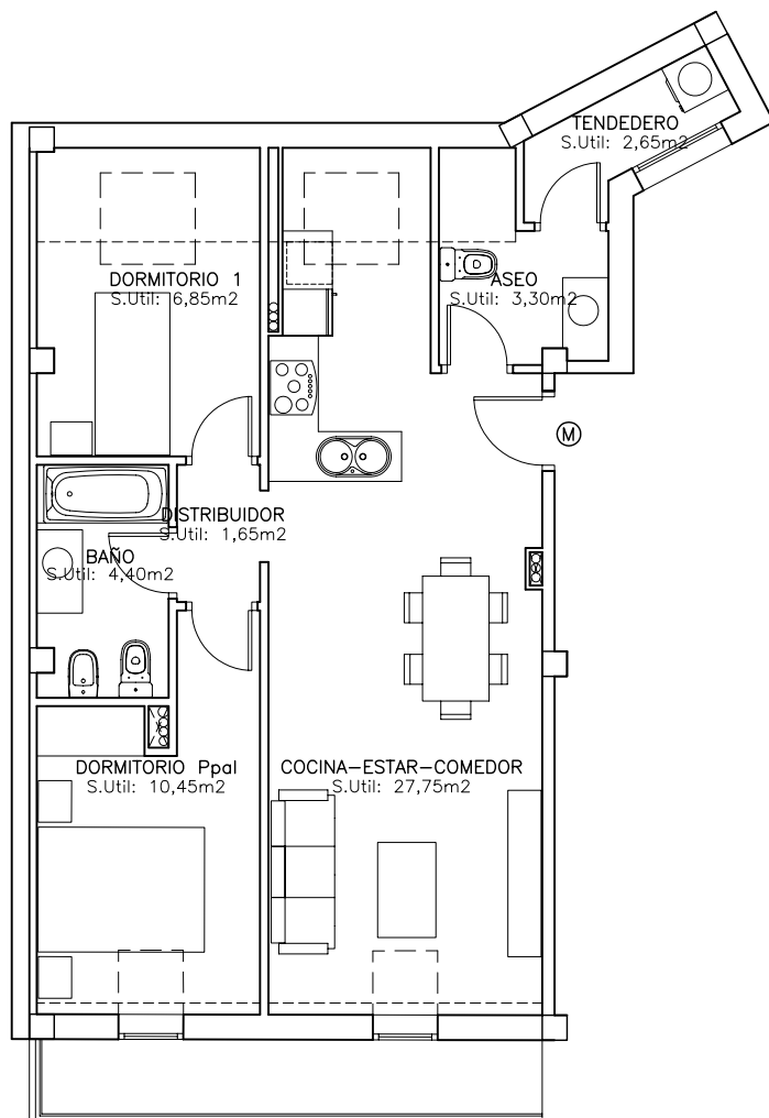
PLANTA BAJOCUBIERTA PORTAL 2 – VIVIENDA M
